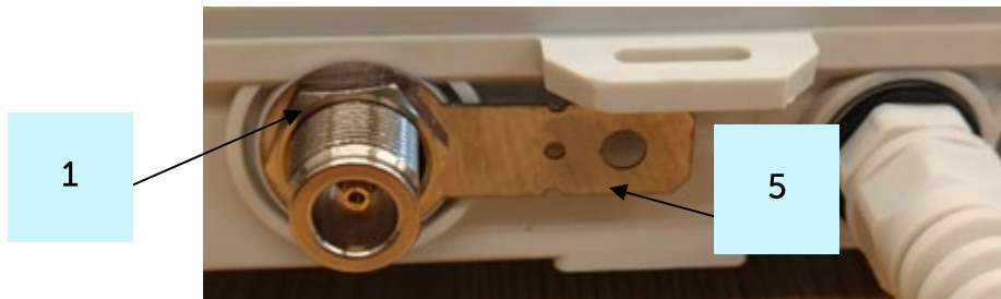
5 – контакт подключения заземления
